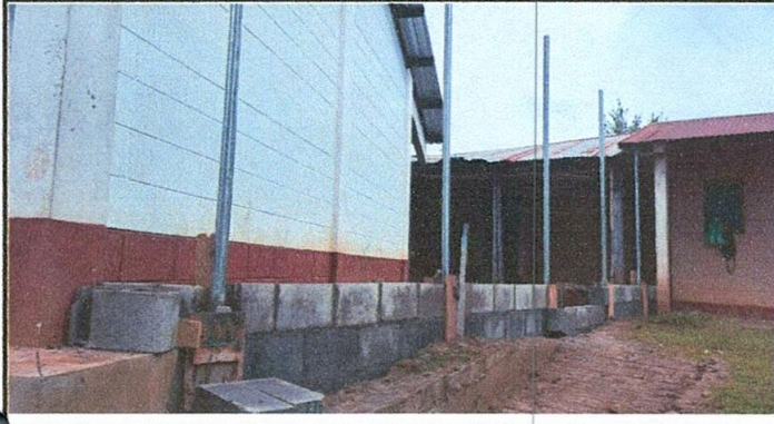
Foto 1: Reparación de muro perimetral de block con tubo y malla galvanizada
